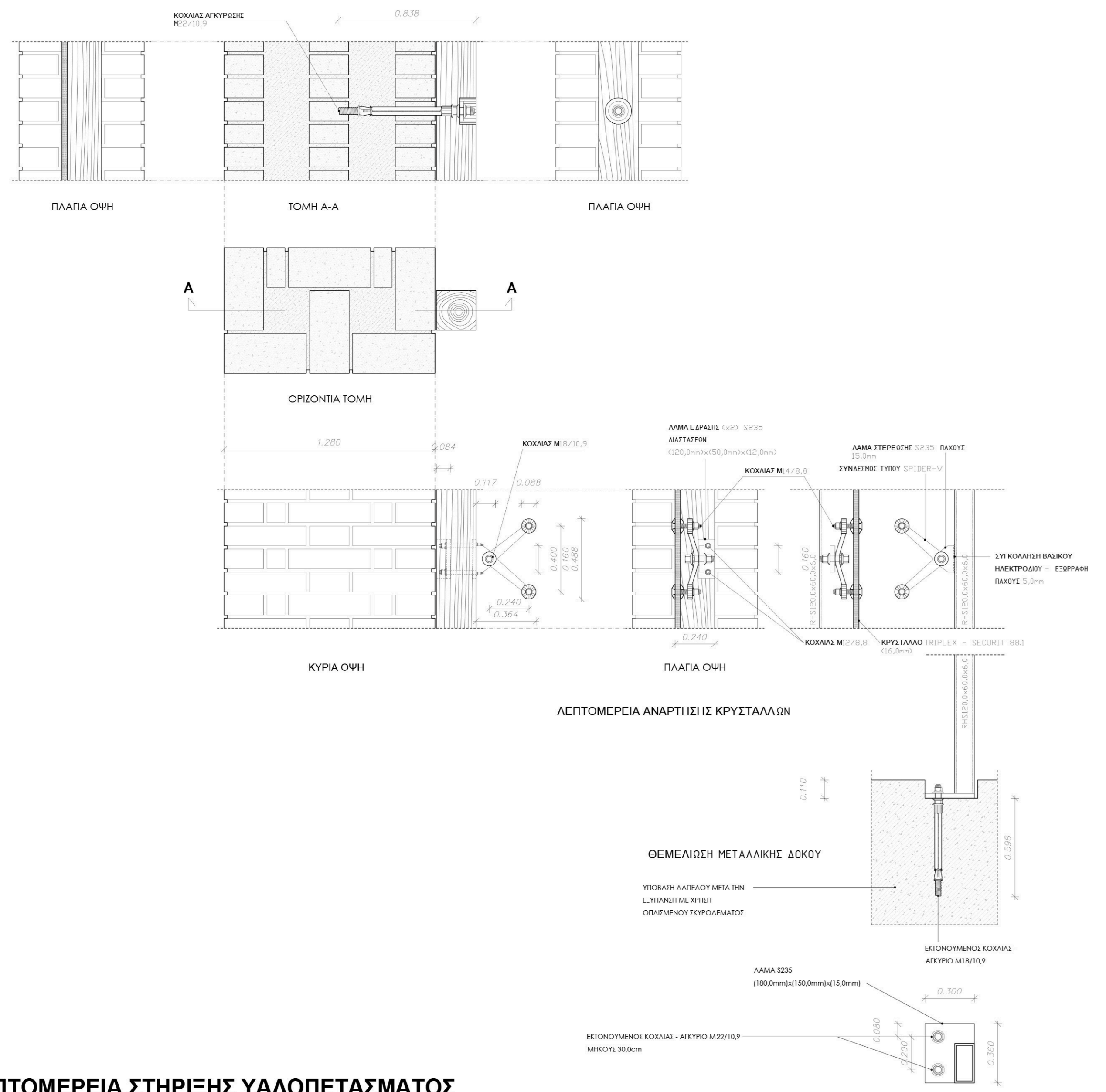
ΛΕΠΤΟΜΕΡΕΙΑ ΣΤΗΡΙΞΗΣ ΥΑΛΟΠΕΤΑΣΜΑΤΟΣ ΚΛΙΜΑΚΑ 1:10
