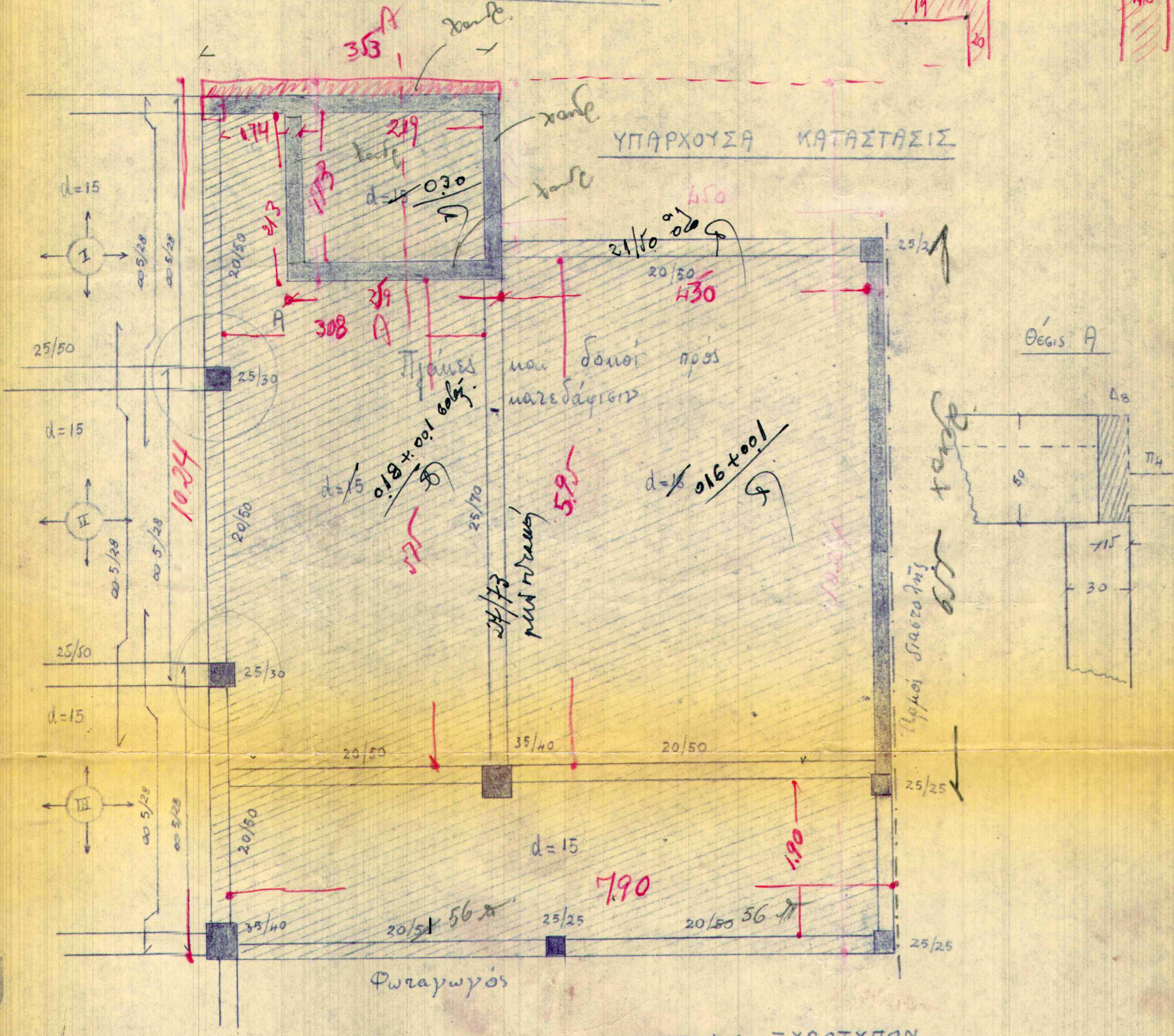
ΚΑΤΟΨΙΣ ΕΥΡΩΤΥΠΩΝ
