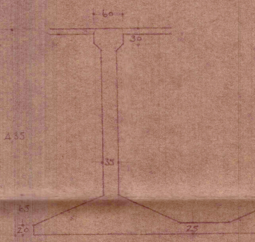
ΤΟΜΗ Γ-Δ
